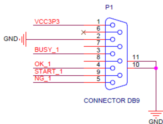
图 2-3: DB9 信号图
