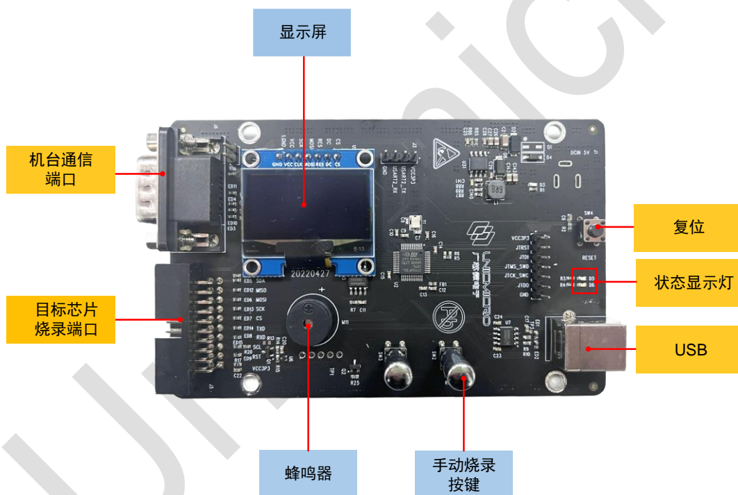
图 1-1: RF 烧录器 EVB 板介绍
