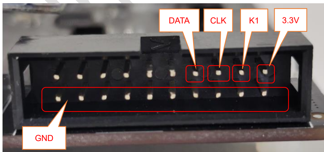
图 2-1: 目标芯片接口
