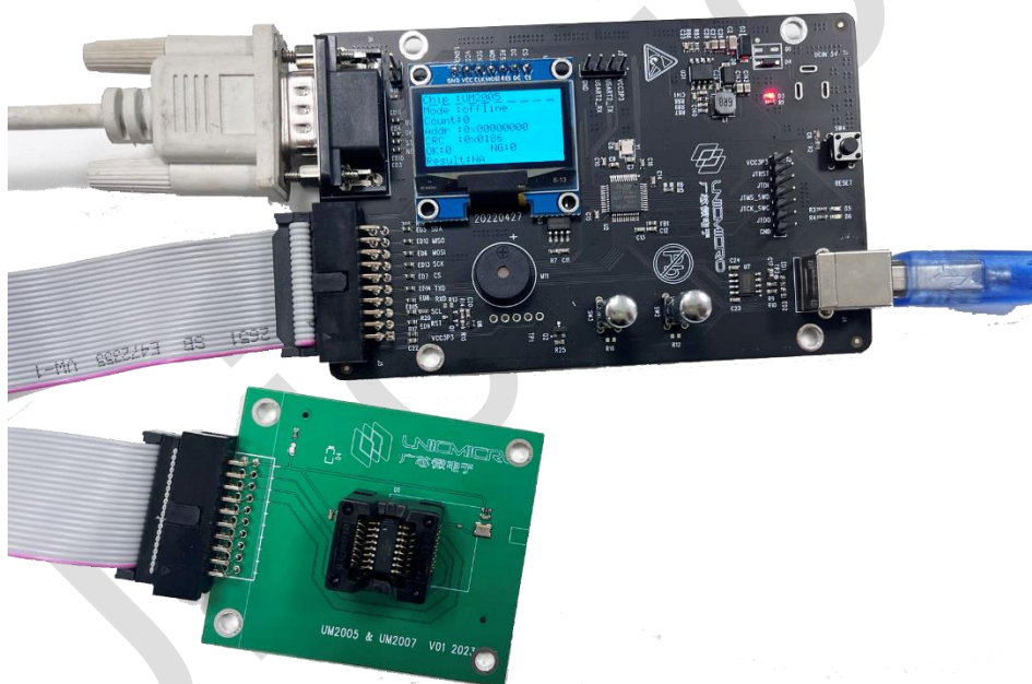
图 2-5：Demo 连接参考
