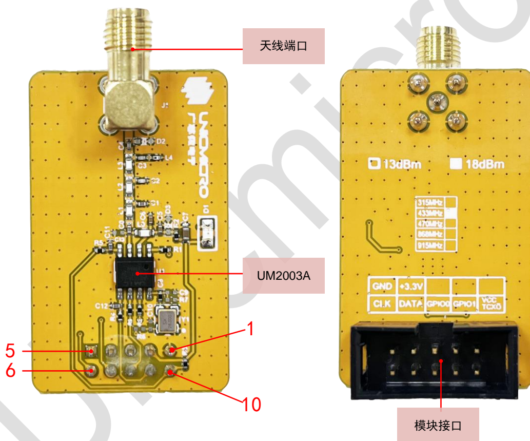
图 2-2: RF-EVB 子板
