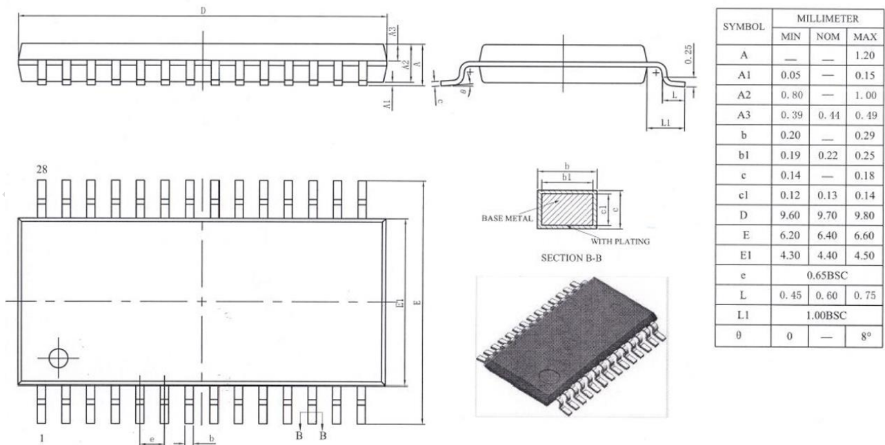
图 5-5: TSSOP28 封装图
