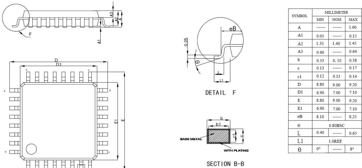
图 5-4: LQFP32 封装图
