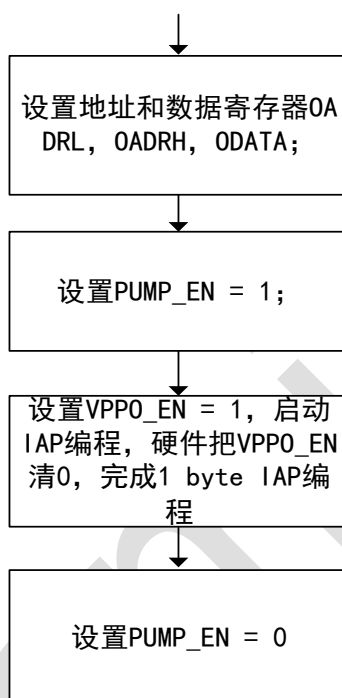
图 5-1: 写操作流程
