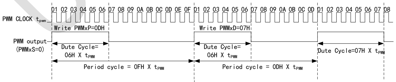
图 6-2: PWM 输出周期或占空比改变范例
