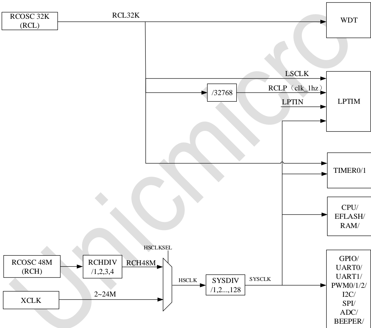
图 4-1: 时钟结构图
