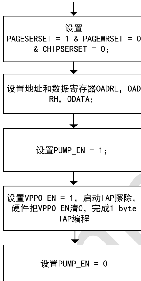
图 5-2: 擦除操作流程
