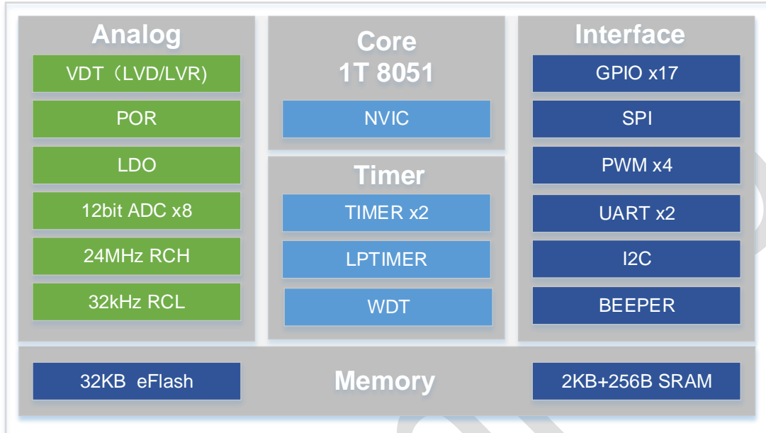
图 1-1：芯片功能图
