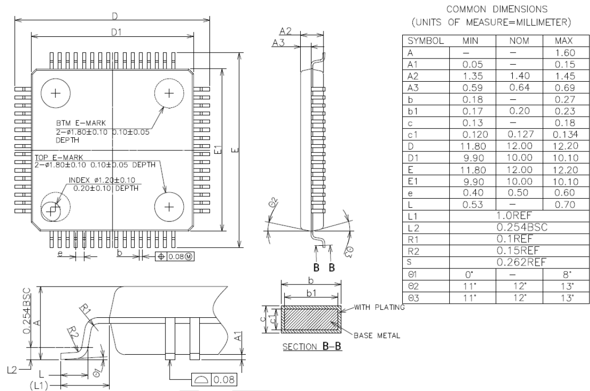
图 5-1: LQFP64 (10*10mm) 封装尺寸图
